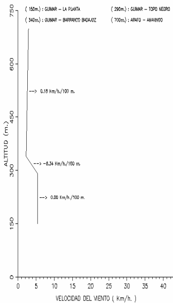
PERFIL VERTICAL – 4/NOVIEMBRE /2006 (13 h.)
