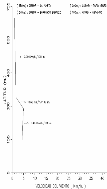
PERFIL VERTICAL – 4/NOVIEMBRE /2006 (17 h.)
