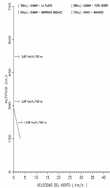
PERFIL VERTICAL – 4/NOVIEMBRE /2006 (21 h.)
