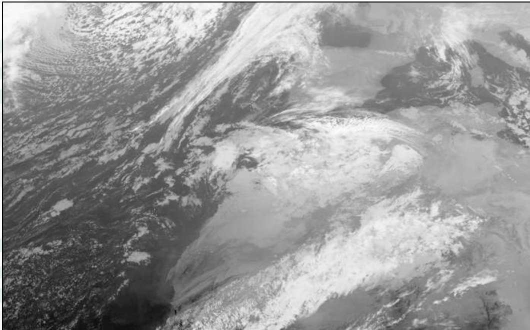
Imagen del satélite Meteosat 8 (infrarrojo): 12 de enero a las 18 h UTC
