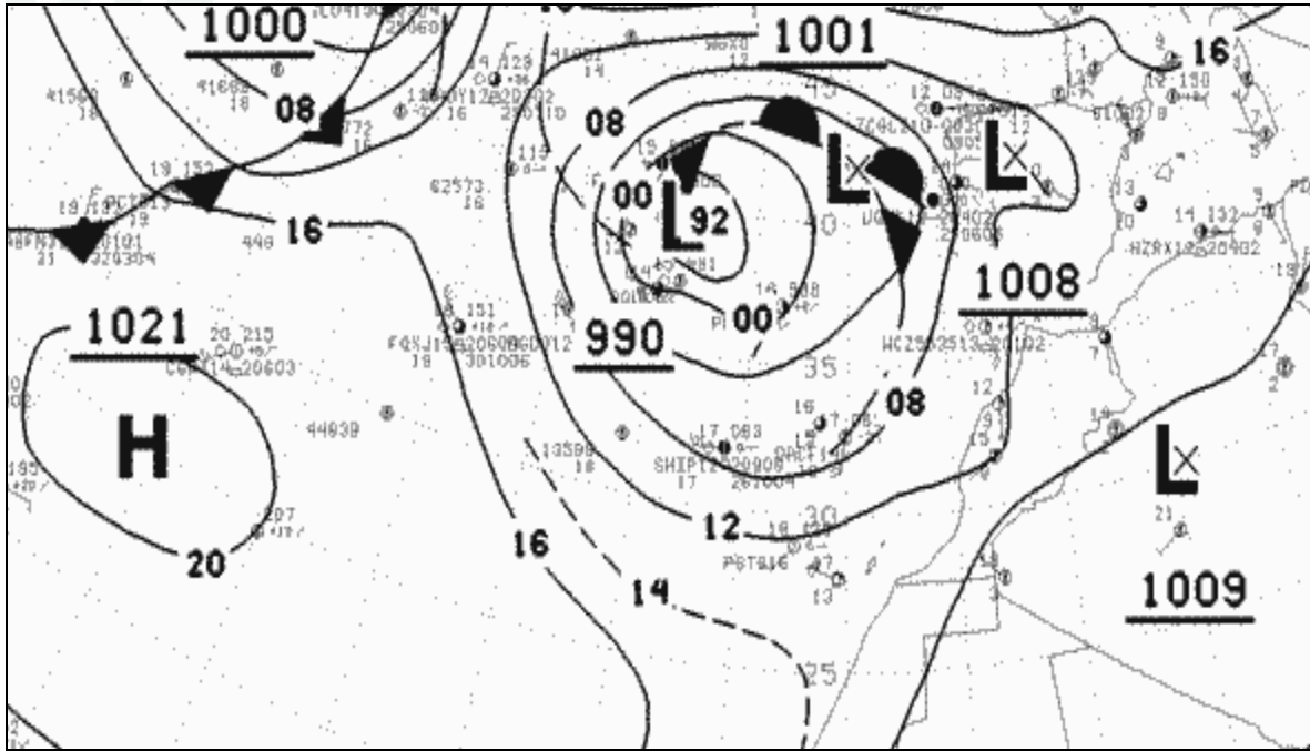
Situación sinóptica: 17 de marzo a las 0 h UTC
