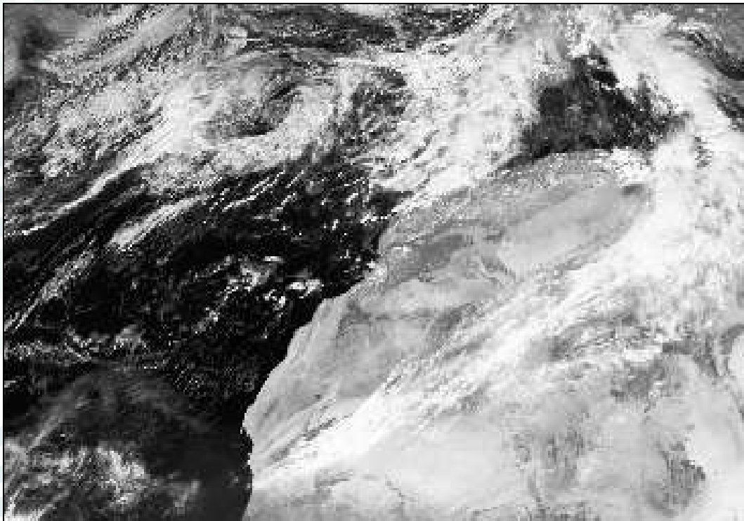
Imagen del satélite Meteosat 8 (visible): 19 de octubre a las 12 h UTC
