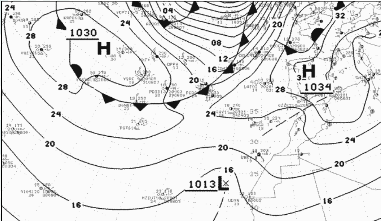
Situación sinóptica: 12 de enero a 0 h TC
