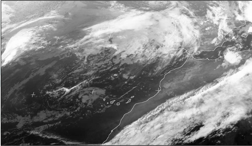
Imagen del satélite Meteosat 8 (infrarrojo): 19 de octubre a las 0 h UTC
