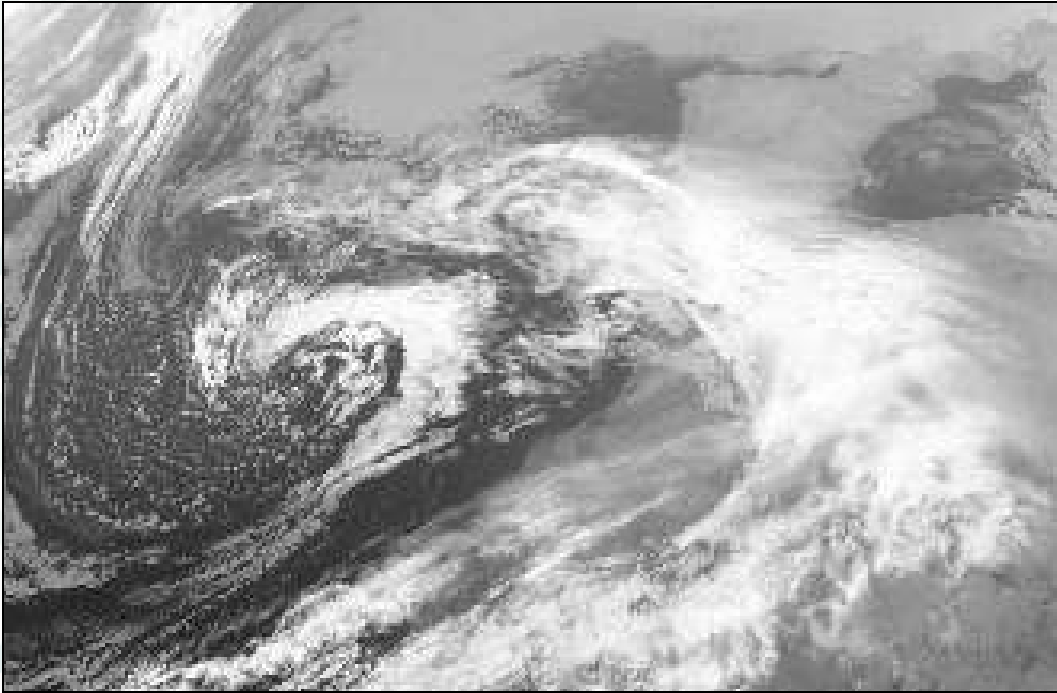
Imagen del satélite Meteosat 8 (infrarrojo): 8 de febrero a las 0 h UTC
