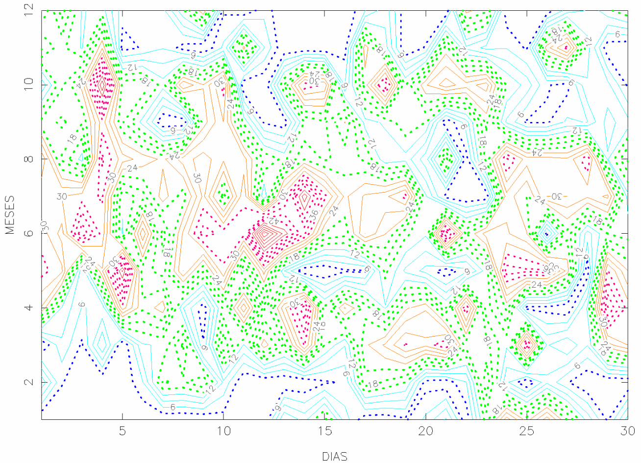
Figura 13: Contorno anual de las frec. relativas de velocidades minutarias menores o iguales a 5 km/h.
