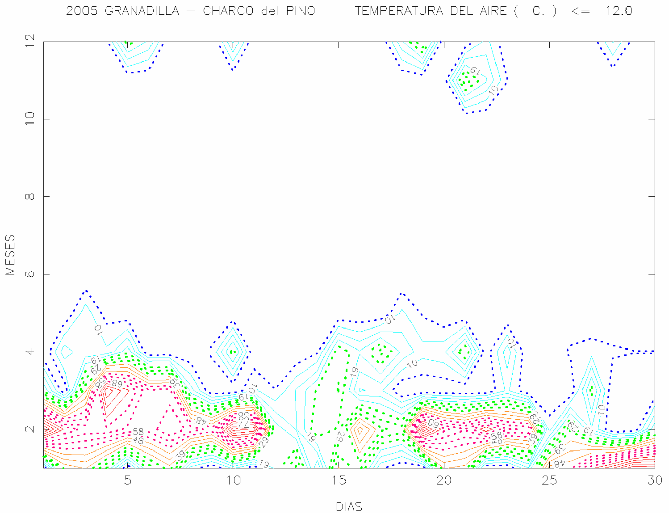
Figura 6: Contorno anual de las frec. relativas de temperaturas minutarías menores o iguales a 12 °C.
