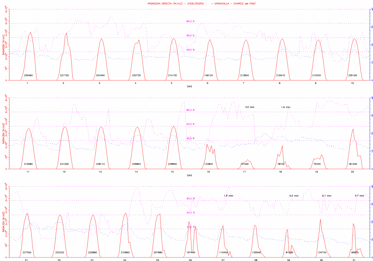
Figura 19: Radiaciones directas horarias y sus relaciones con otras variables en ENERO.
