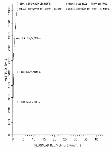
PERFIL VERTICAL - 4/NOVIEMBRE /2006 (21 h.)
