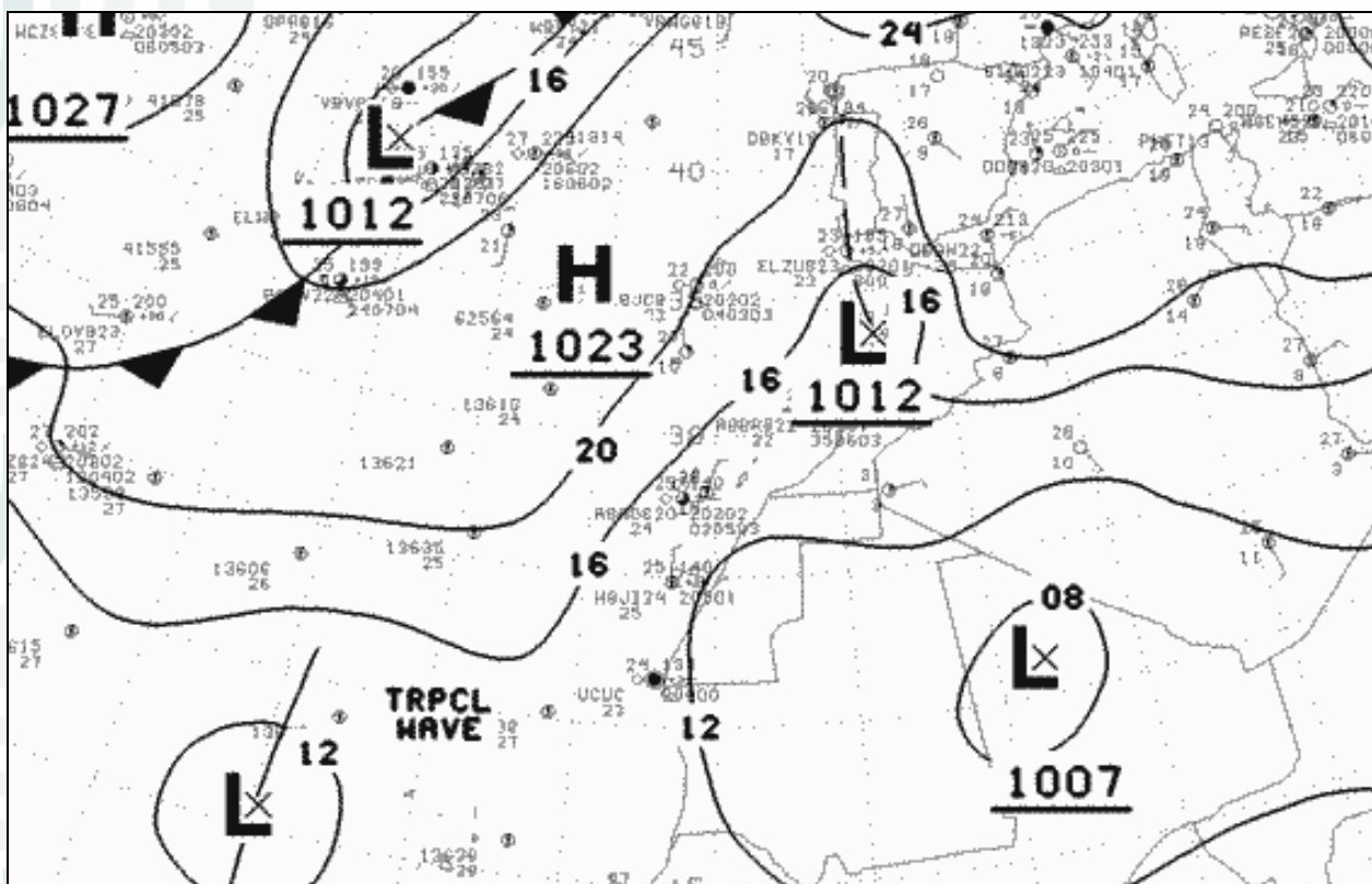
Situación sinótica: 5 de septiembre a las 0 h UTC
