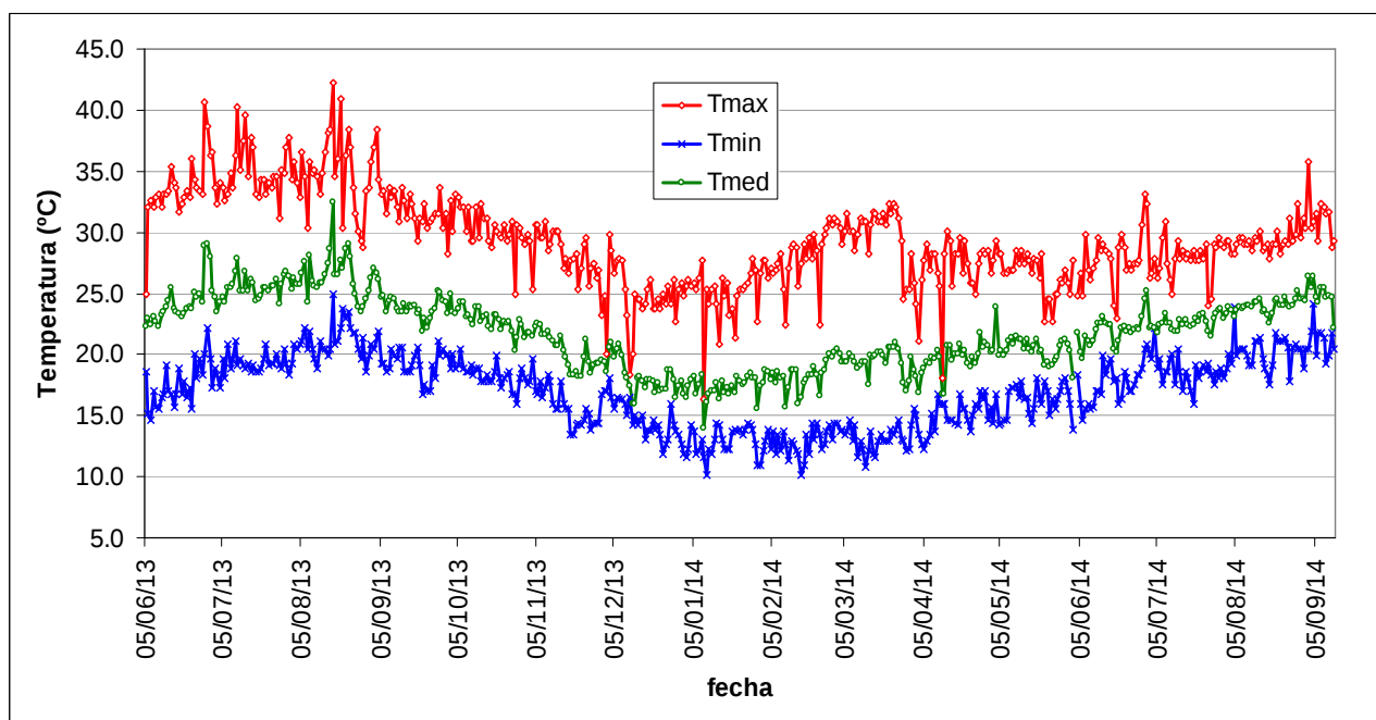
Figura 3: Temperaturas registradas en el invernadero del ensayo del Sur
