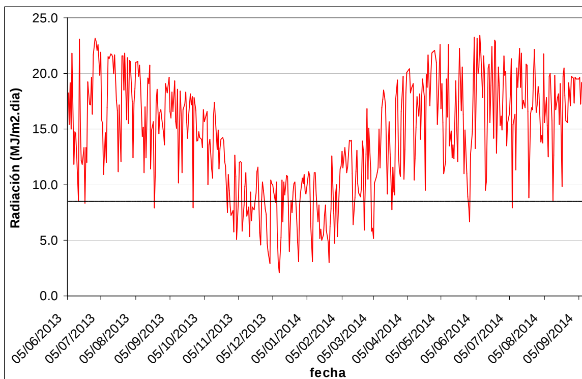
Figura 2: Radiación estimada dentro del invernadero del ensayo del Norte (la recta corresponde al valor límite de 8.5 \text{ MJ/m}^2 \cdot \text{día} ).
