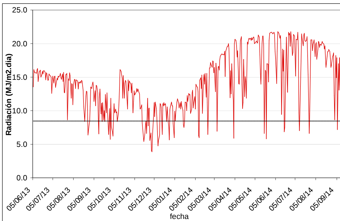
Figura 1: Radiación estimada dentro del invernadero del ensayo del Sur (la recta corresponde al valor límite de 8.5 \text{ MJ/m}^2 \cdot \text{día} ).
