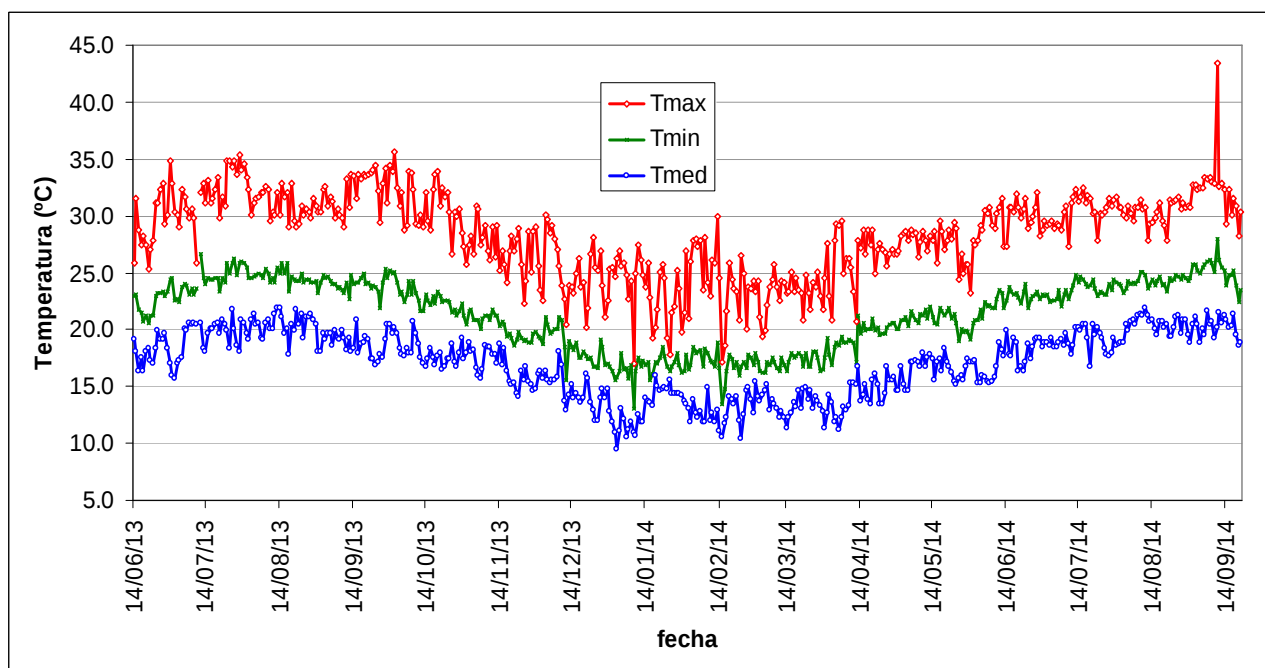
Figura 4: Temperaturas registradas en el invernadero del ensayo del Norte.
